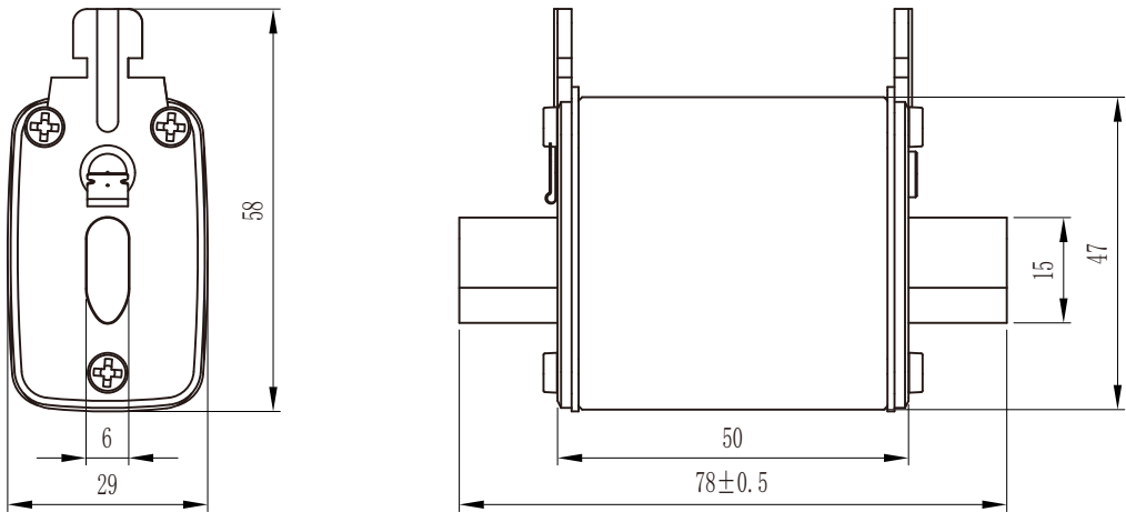
RT16-00(NT00、NH00) 外形、及安装尺寸 (mm)
