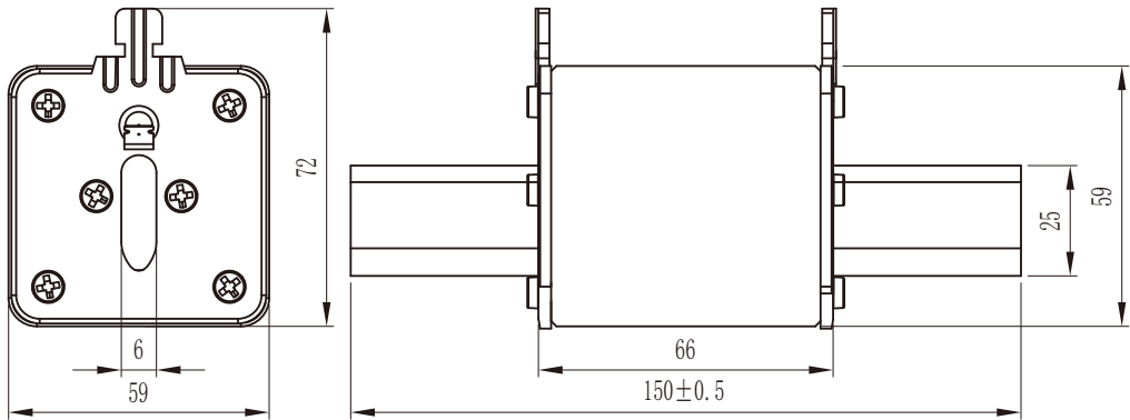
RT16-2(NT2、NH2) 外形、及安装尺寸 (mm)
