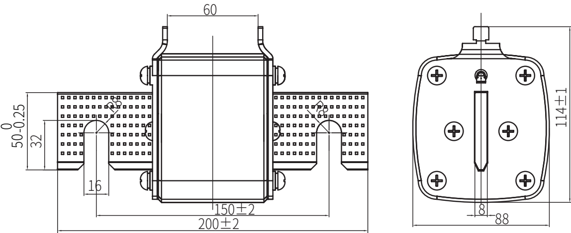
NT4(NH4) 外形、及安装尺寸 (mm)
